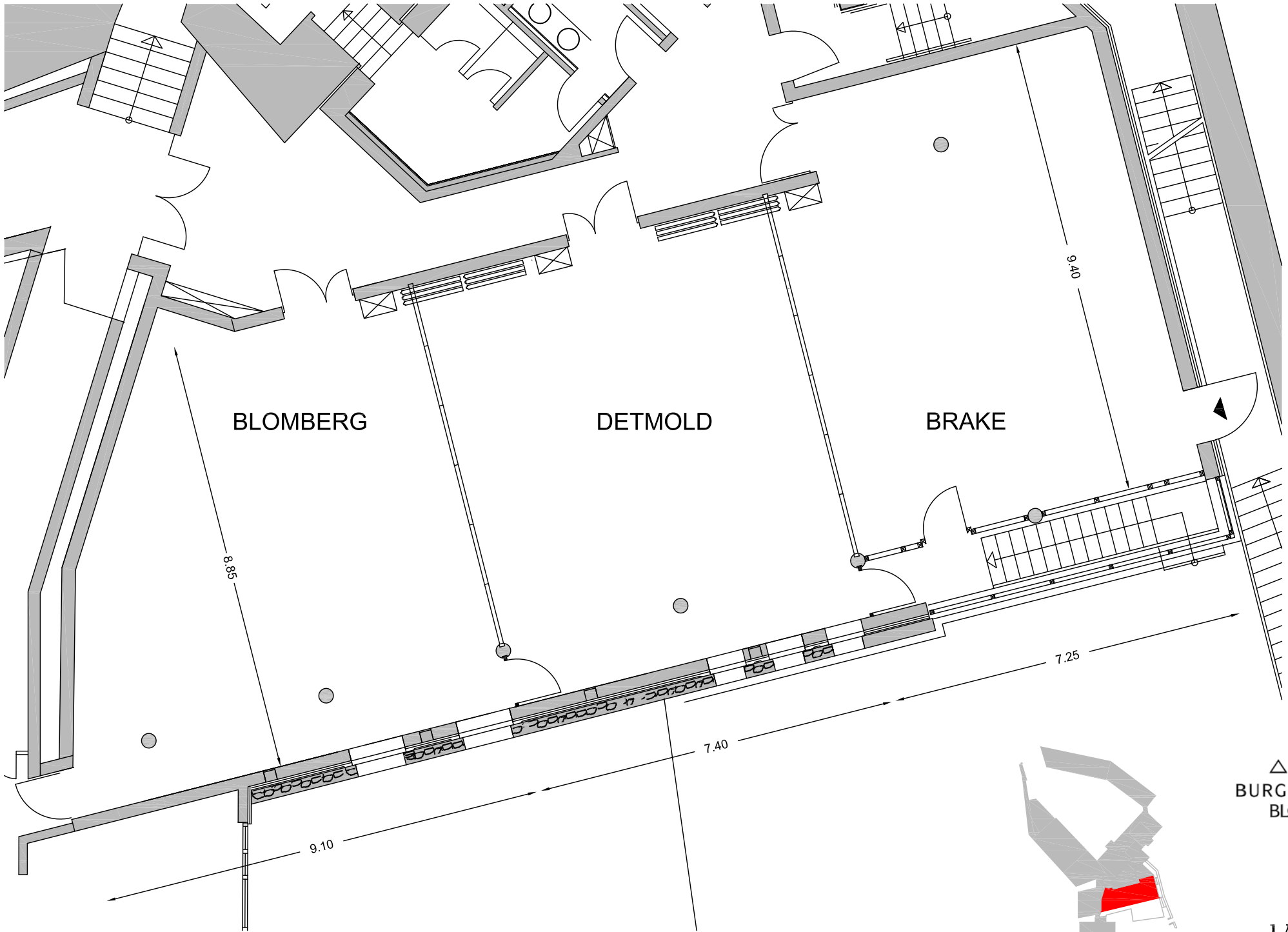
NEUER TAGUNGSTRAKT. GRUNDRISS 1.100
